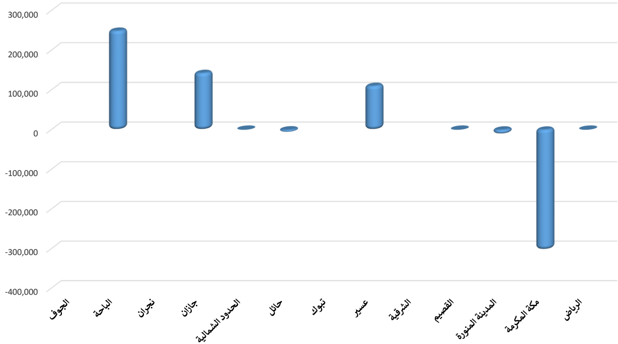
مقدار التغير في حجم تخزين السدود (م ٣ ) بين يومي الثلاثاء ١٠/١٠/١٤٤٤هـ والاربعاء ١١/١٠/١٤٤٤هـ
